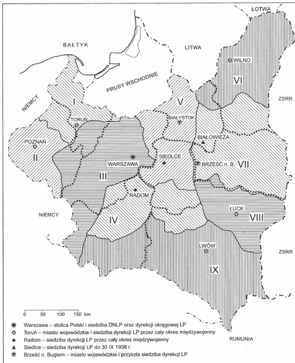
Ryc. 2. Okręgi dyrekcyjne lasów państwowych sprzed 1 X 1938 r. Linie kropkowane oznaczają nowe granice dyrekcji od 1 X 1938 r. (J. Broda: „Historia leśnictwa w Polsce”, Poznań 2000)
